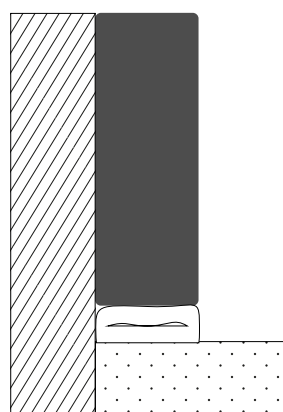
2 Ecrasement du joint mécanique
