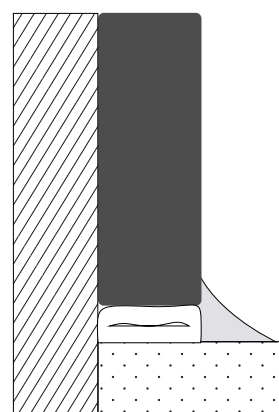
3 Finition avec un joint de silicone
